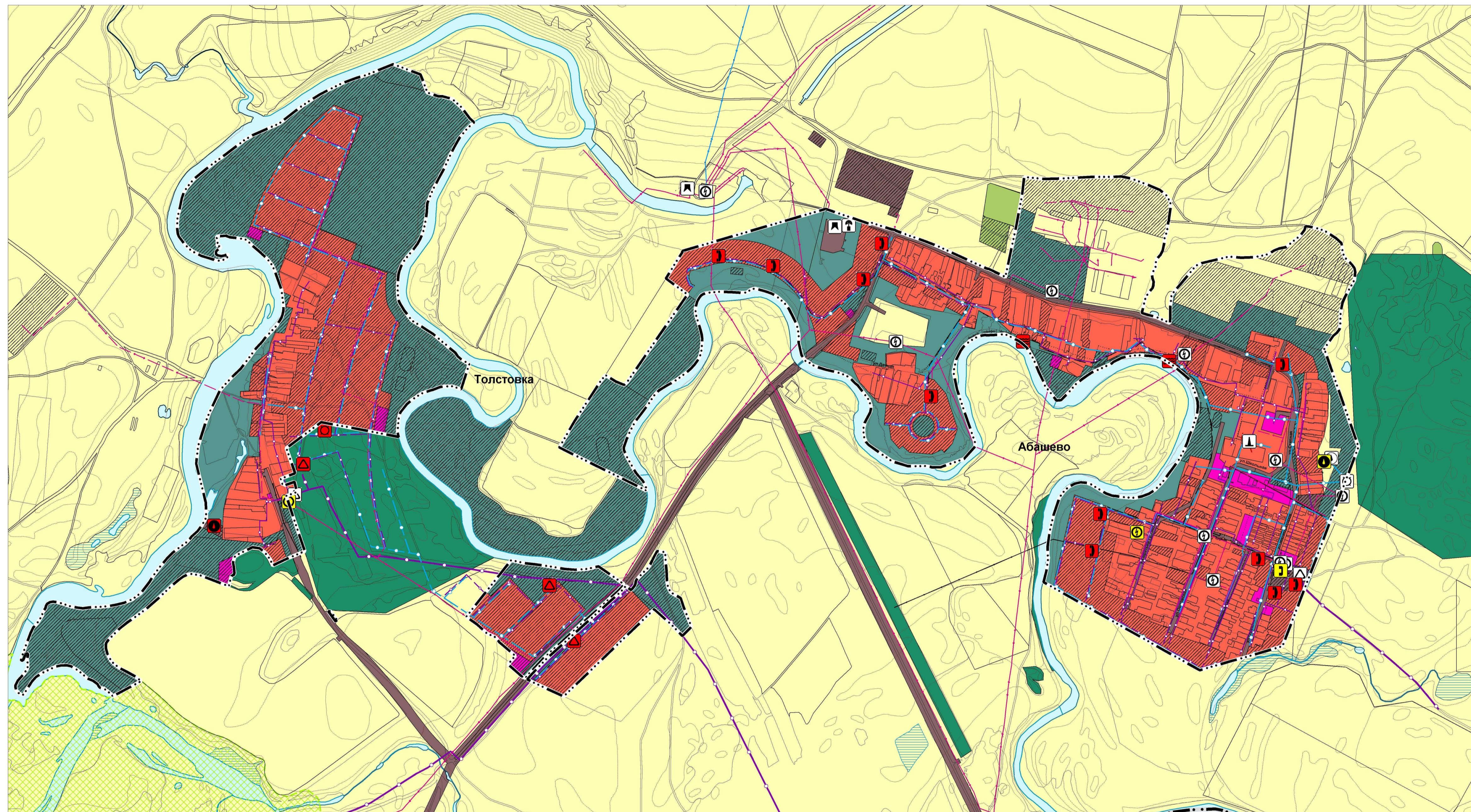
Карта планируемого размещения объектов инженерной инфраструктуры местного значения с. Орловка муниципального района Хворостянский Самарской области
