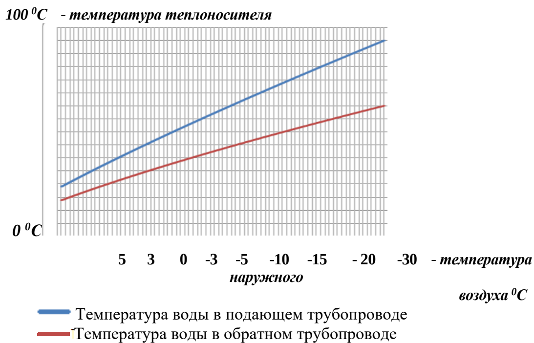
Рис. № 4 - Температурный график качественного регулирования 95/70 °C
